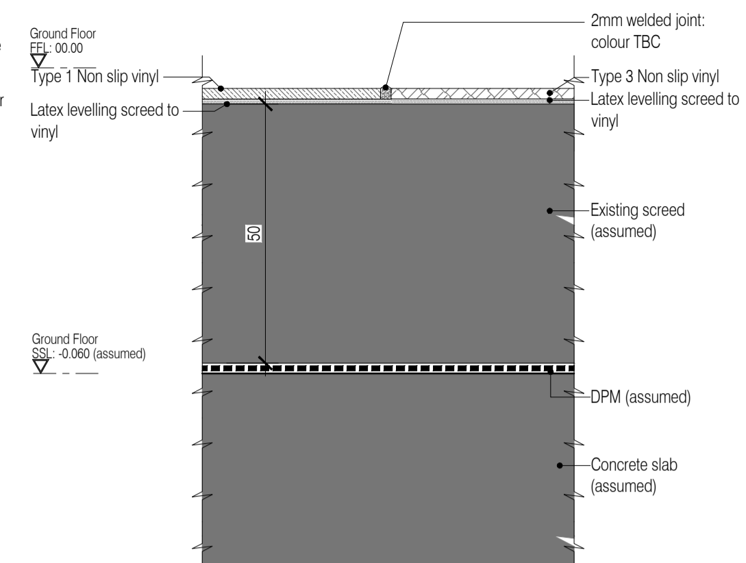
20 Non slip vinyl Type 1 / Non slip vinyl Type 3 Interface Scale:1:1
