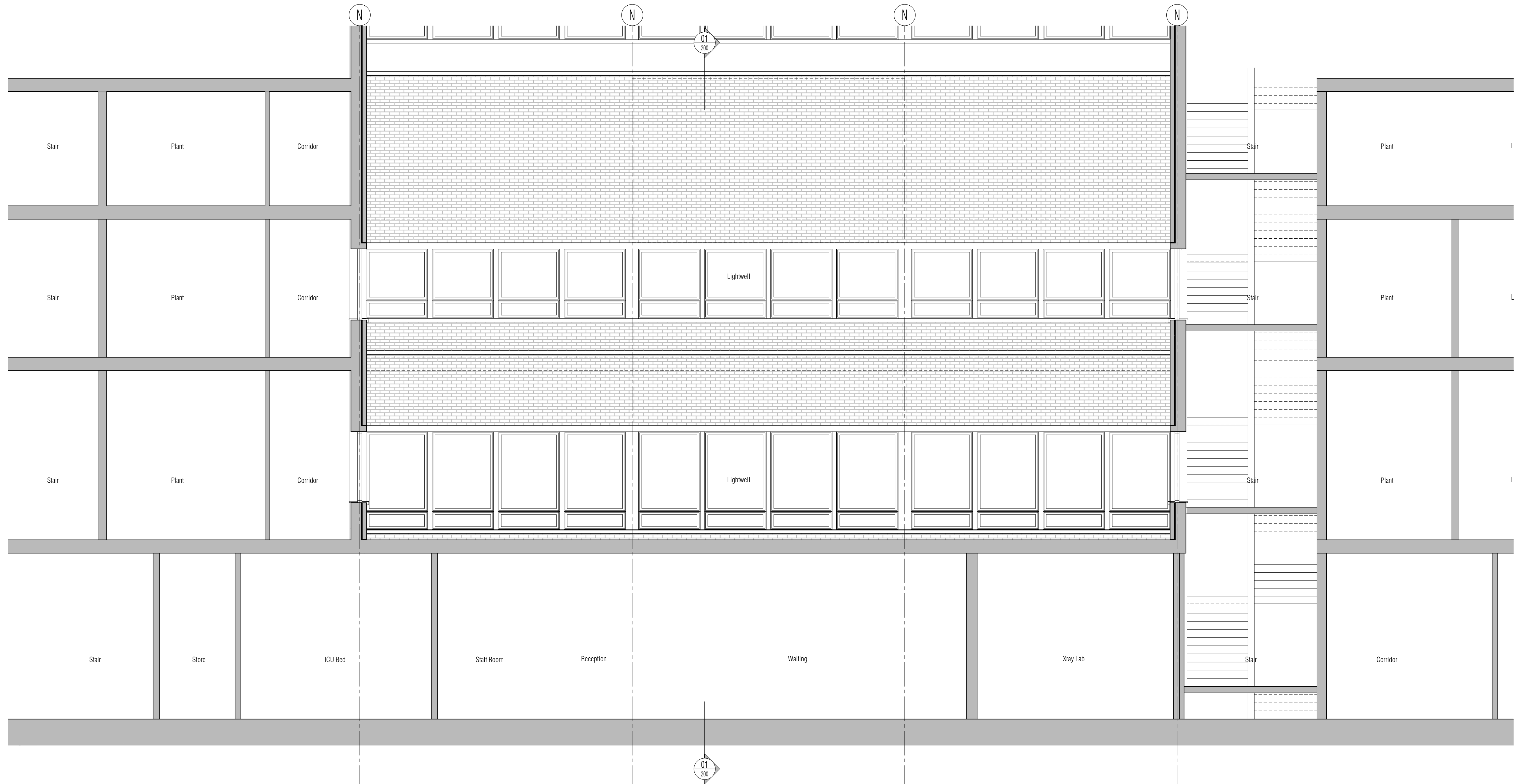
01 Existing Section 06 Scale: 1:50
