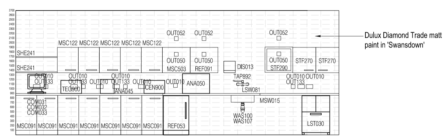
02 Elevation A Scale: 1:50
