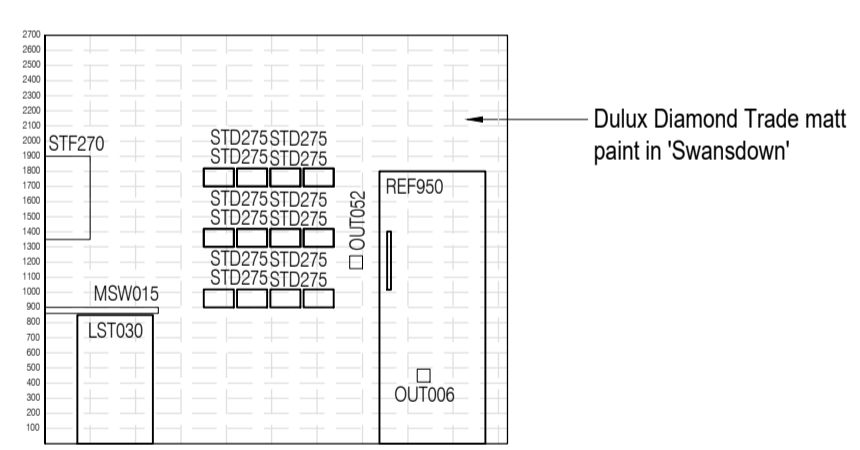
03 Elevation B Scale: 1:50
