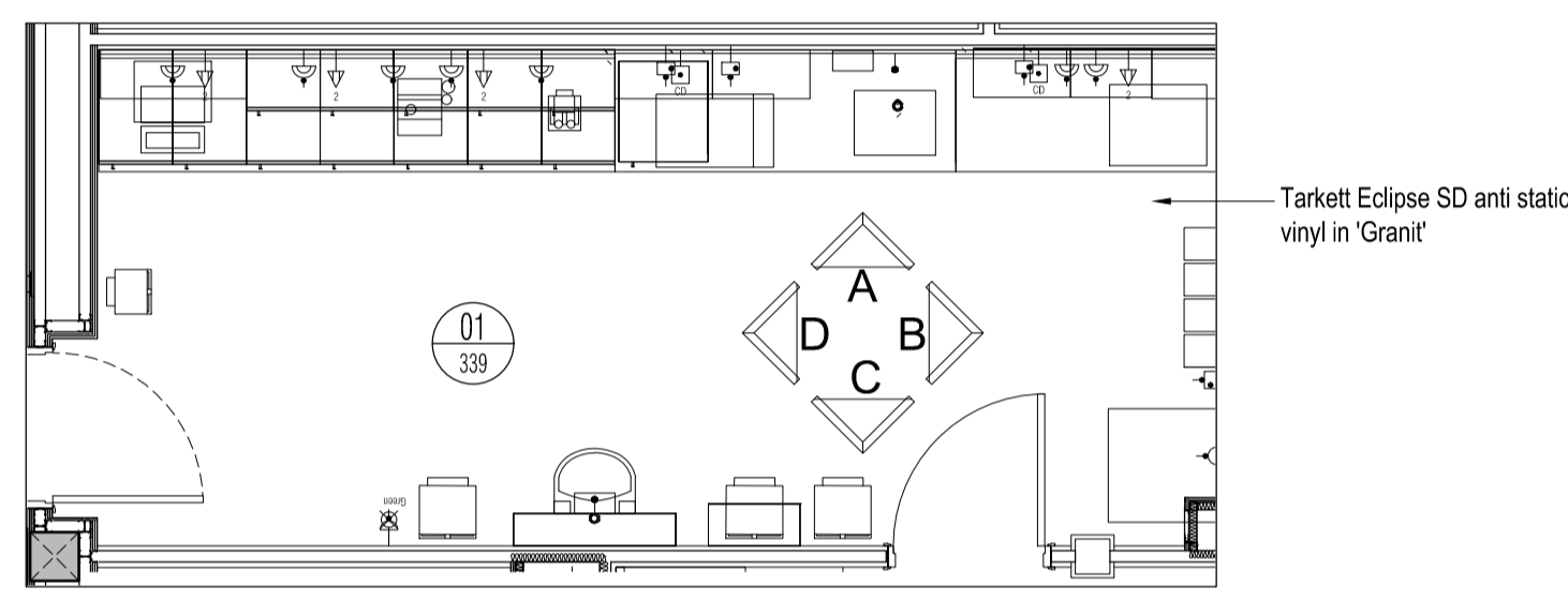
01 Floor Plan Scale: 1:50
