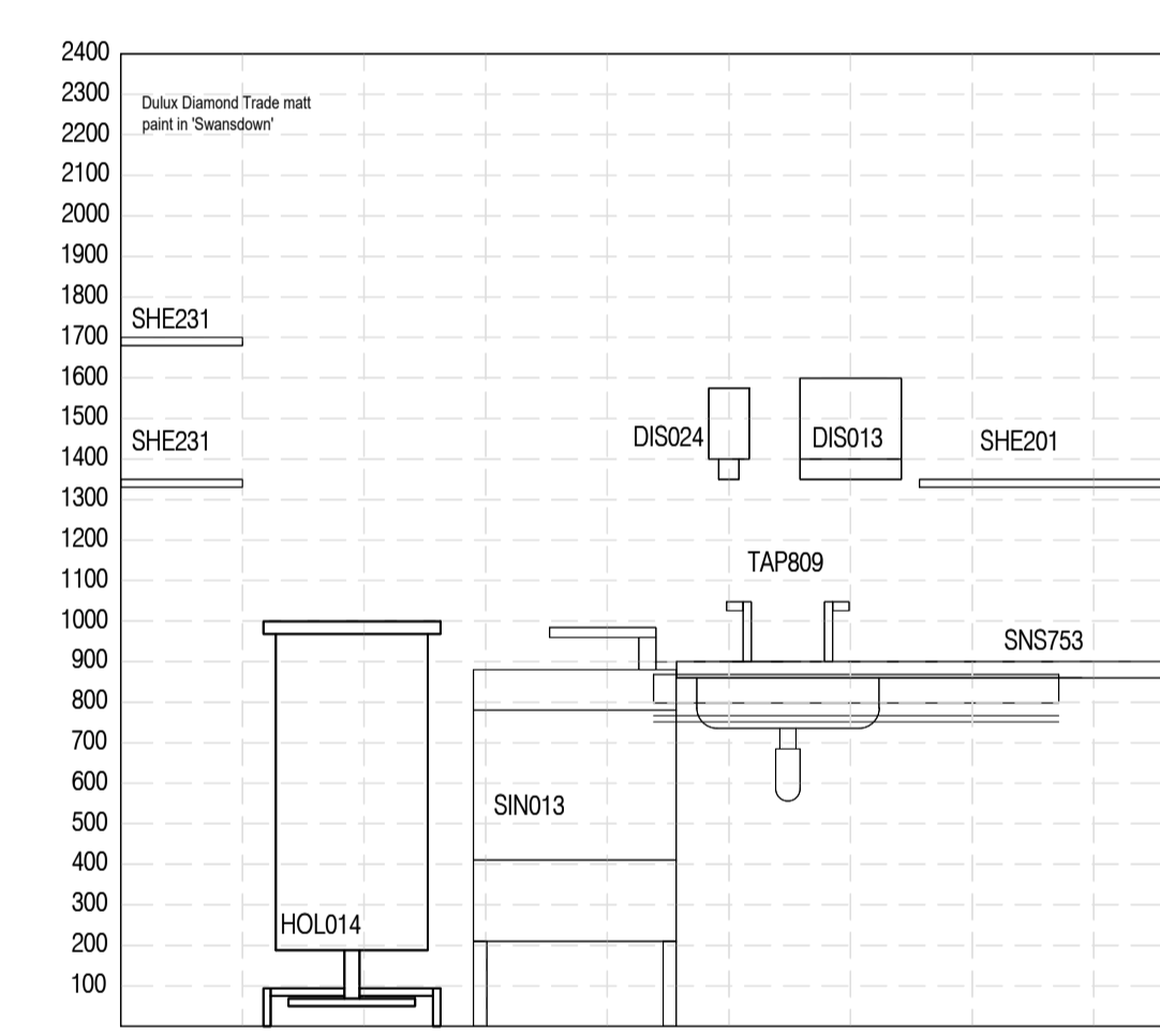
03 Elevation B Scale: 1:20
