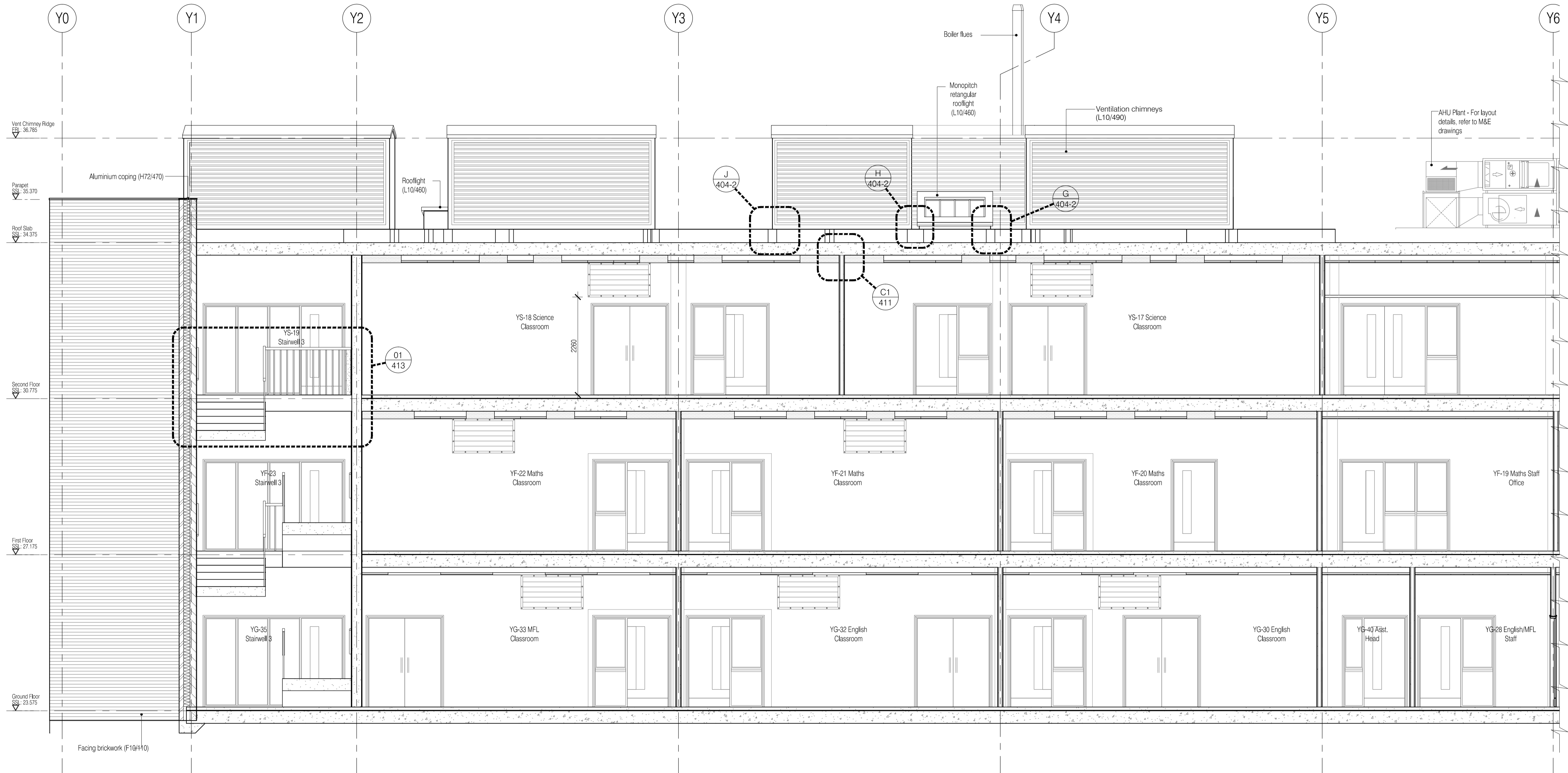
Section C - C Scale: 1:50
