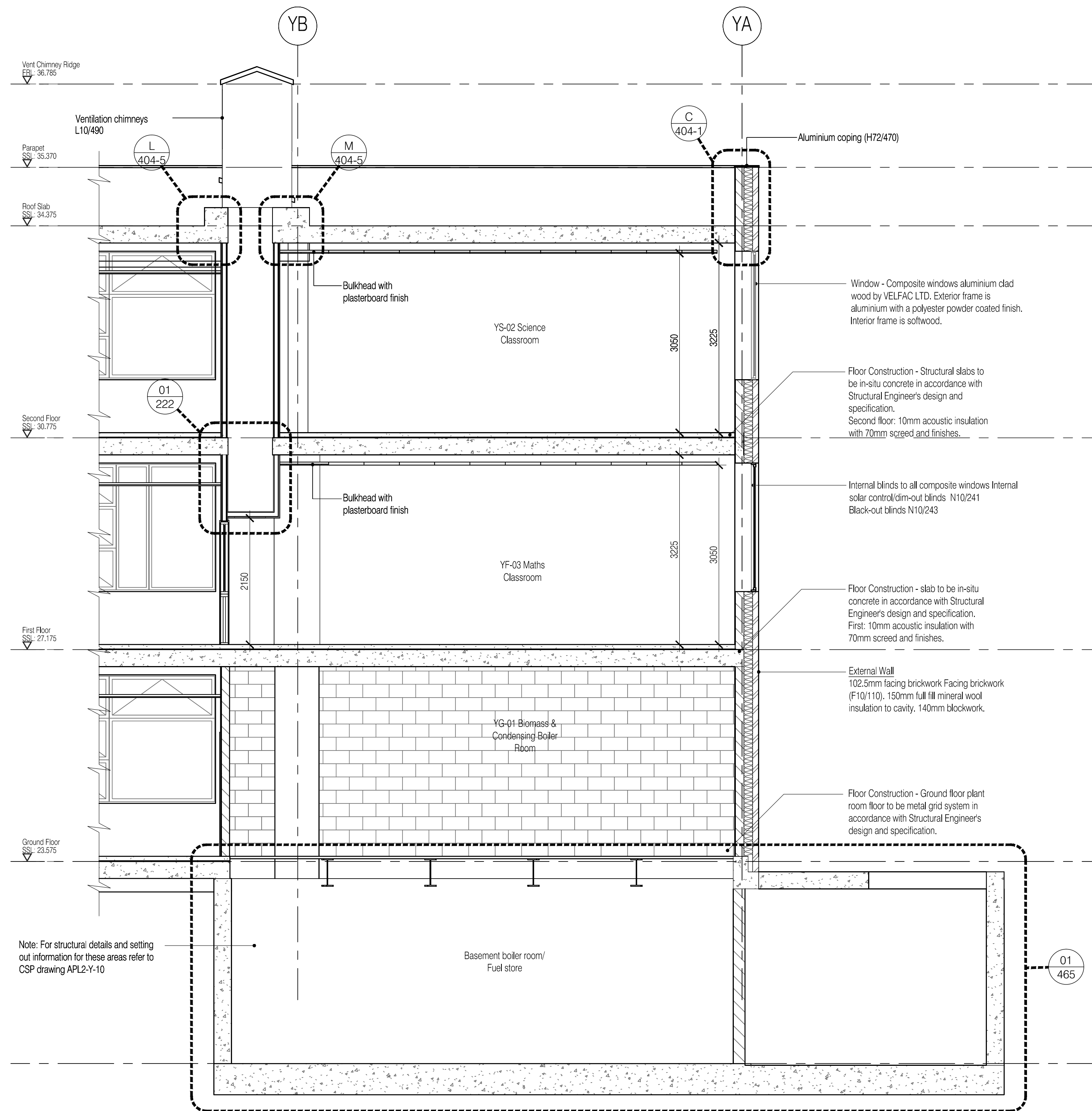
Section D - D Scale: 1:50
