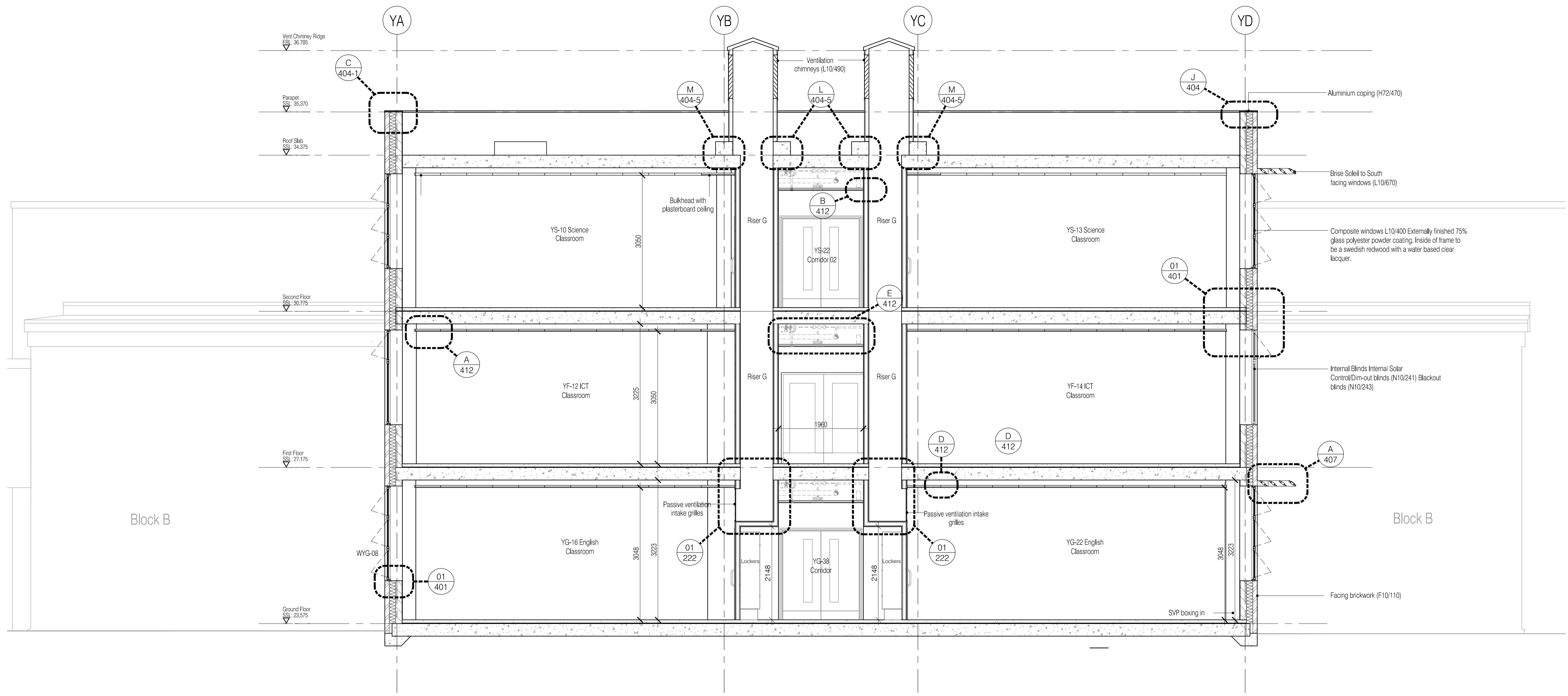
Section F - F Scale: 1:50
