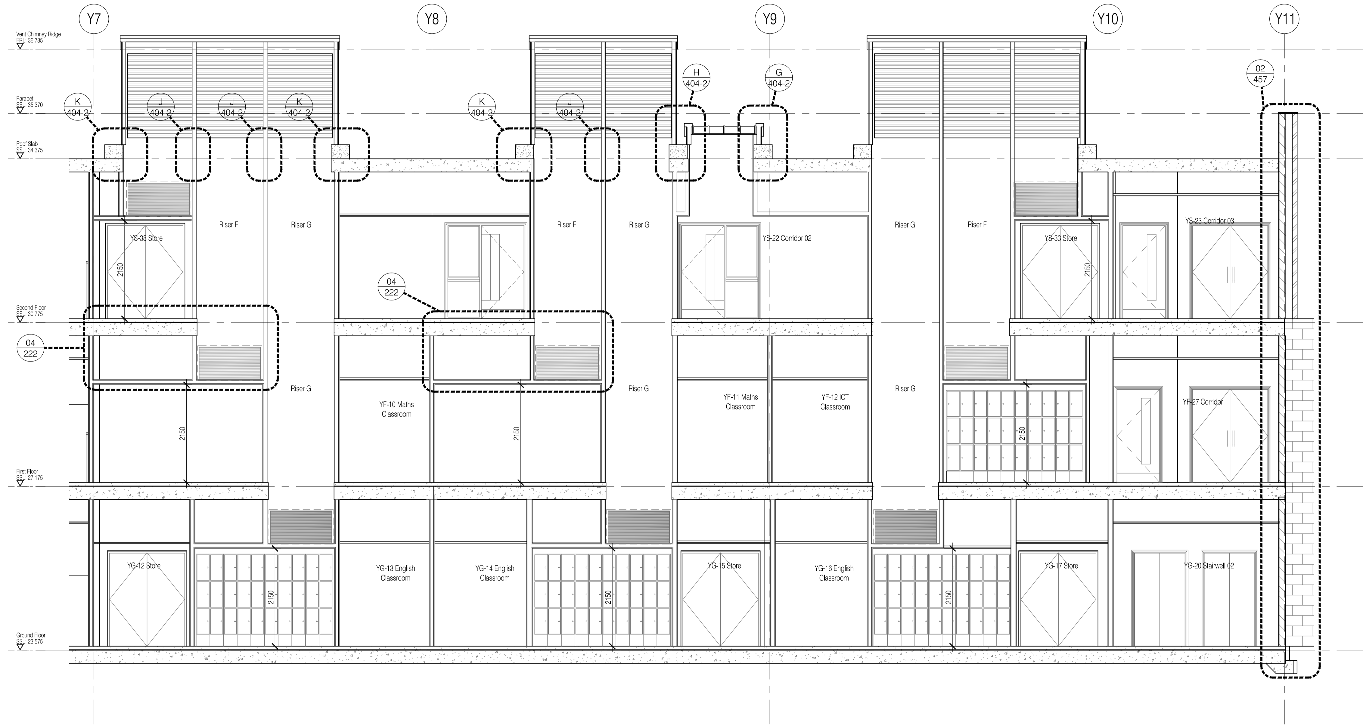
Section L - L Scale: 1:50
