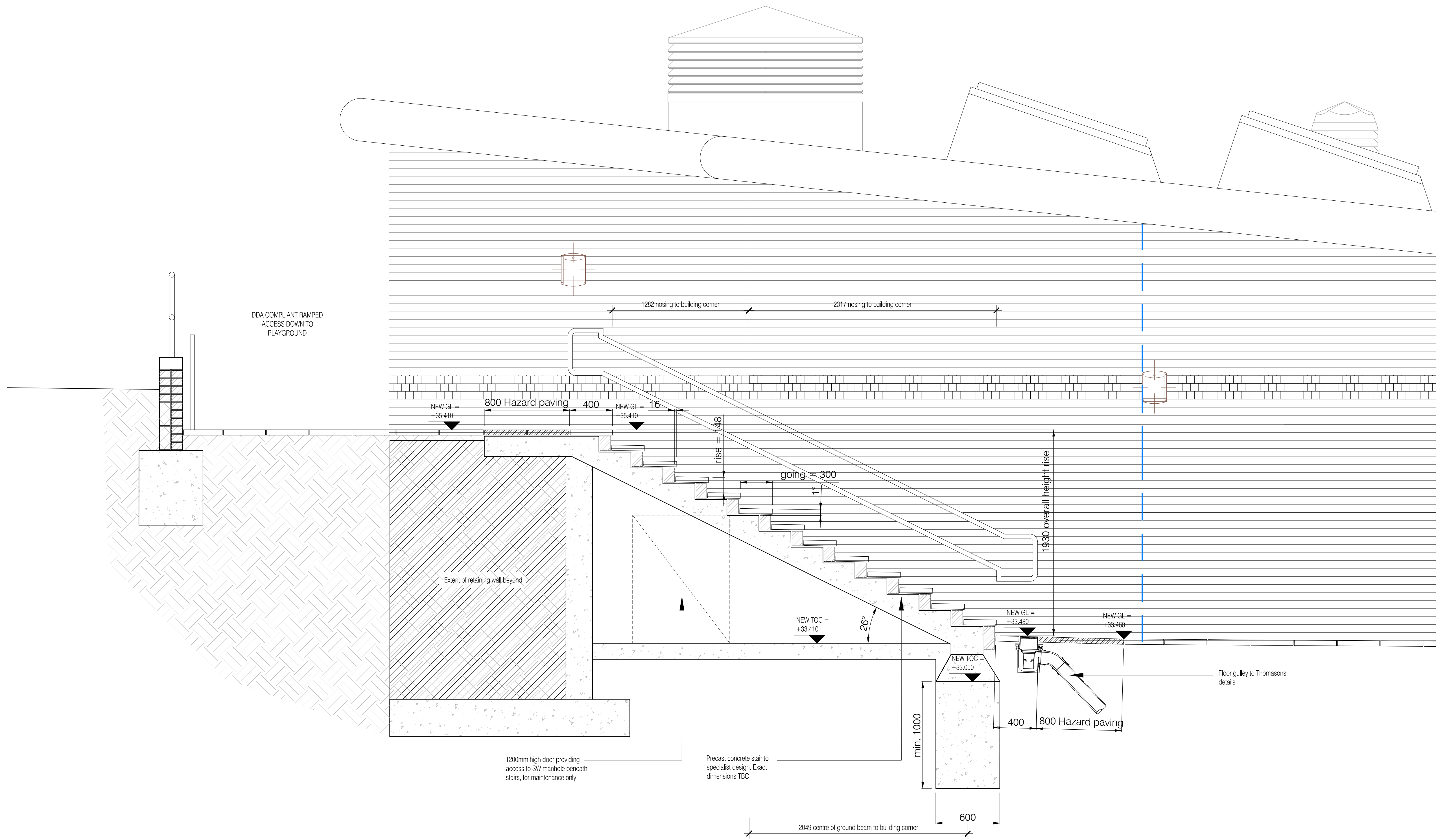
01 External Stair Detail Scale: 1:20
